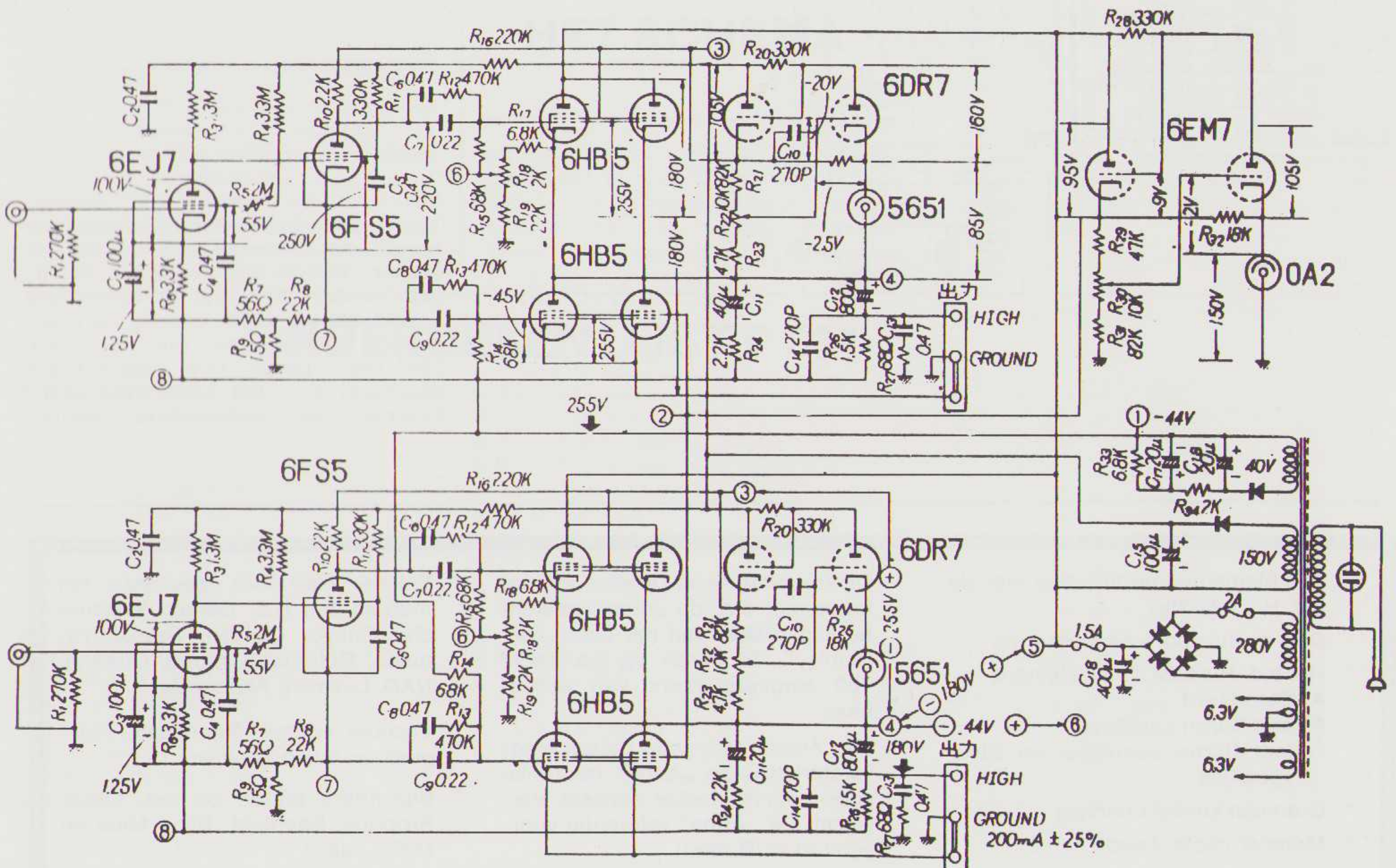
Afb. 11 : De H-3 van Futterman. Hij geeft 30 watt aan 16 ohm bij een bandbreedte van 100 KHz en een vervorming in de orde van 0,2 %
